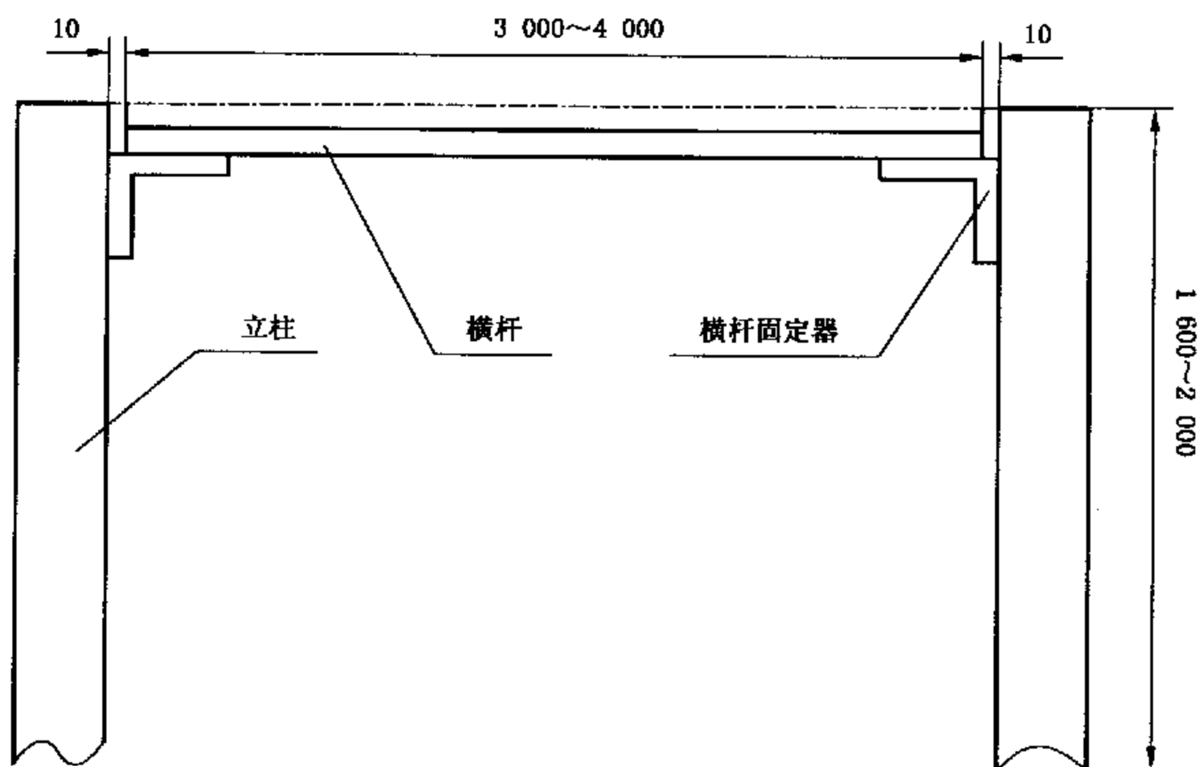
图 1 跳高架示意图
